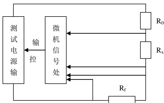
图 1 测量原理示意图
